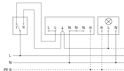
Schaltplan Anschluss über einen Wechselschalter für Dauerlicht- und Automatik-Betrieb
